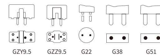
口金
