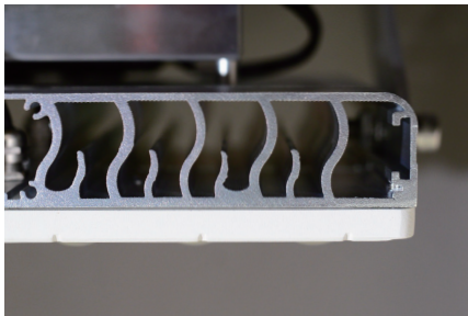
ヒートシンク独自形状による放熱効果アップ
