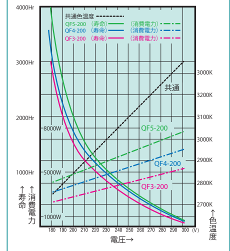
電圧・寿命・色温度・消費電力曲線
