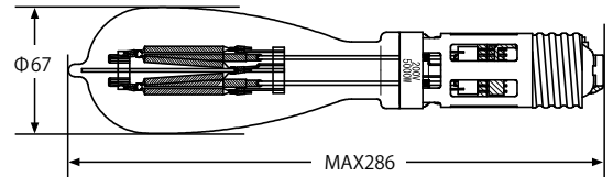
QF5-200
