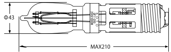
QF1-200
