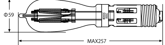
QF3-200
