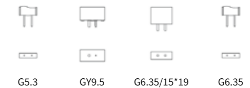
口金
